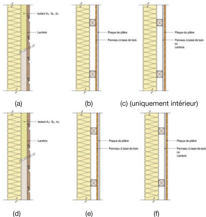
Figure 16 : Montage sur support bois
