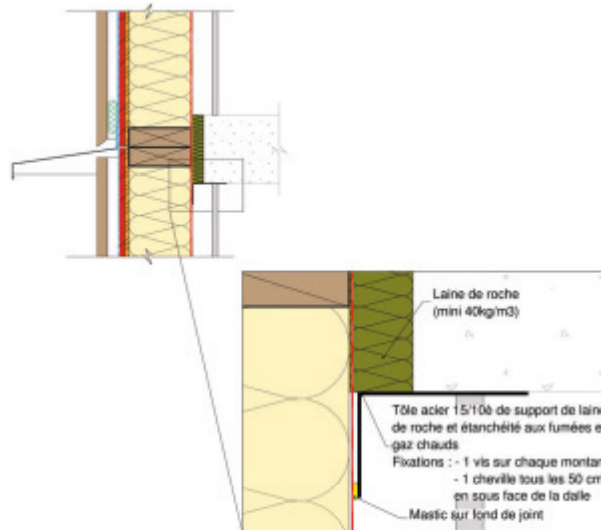
Figure 25 : Traitement de l'étanchéité au nez de dalle béton (si la durée de résistance au feu de la structure est inférieure ou égale à 90 minutes)
