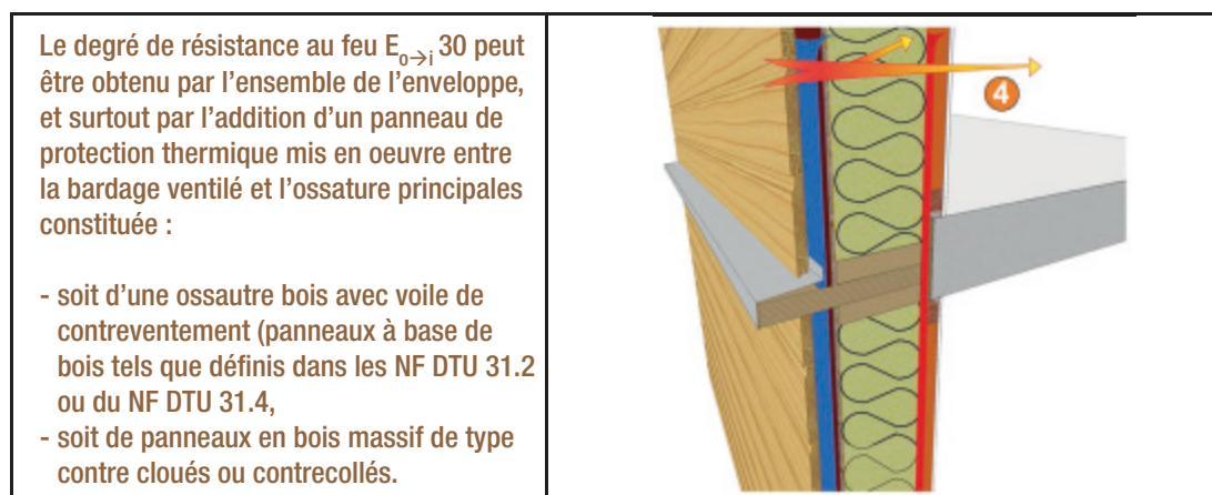
Figure 21 : Représentation de l'exigence feu côté parement extérieur
