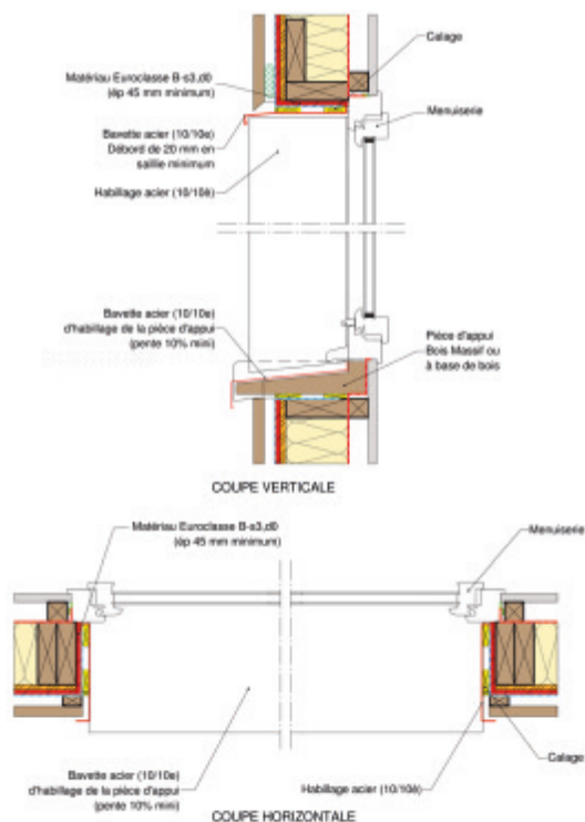
Figure 33 : Traitement des embrasures de menuiseries avec un matériau A2-s3, d0 + habillage acier
