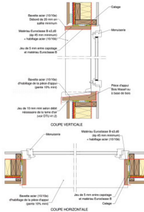
Figure 32 : Traitement des embrasures de menuiseries avec un matériau B-s3, d0 + habillage acier
